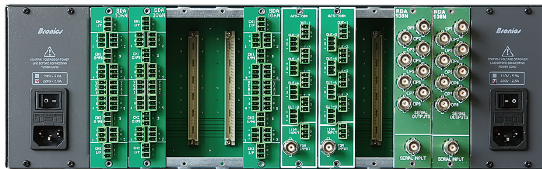
Rear View(Module 장착된 상태)
